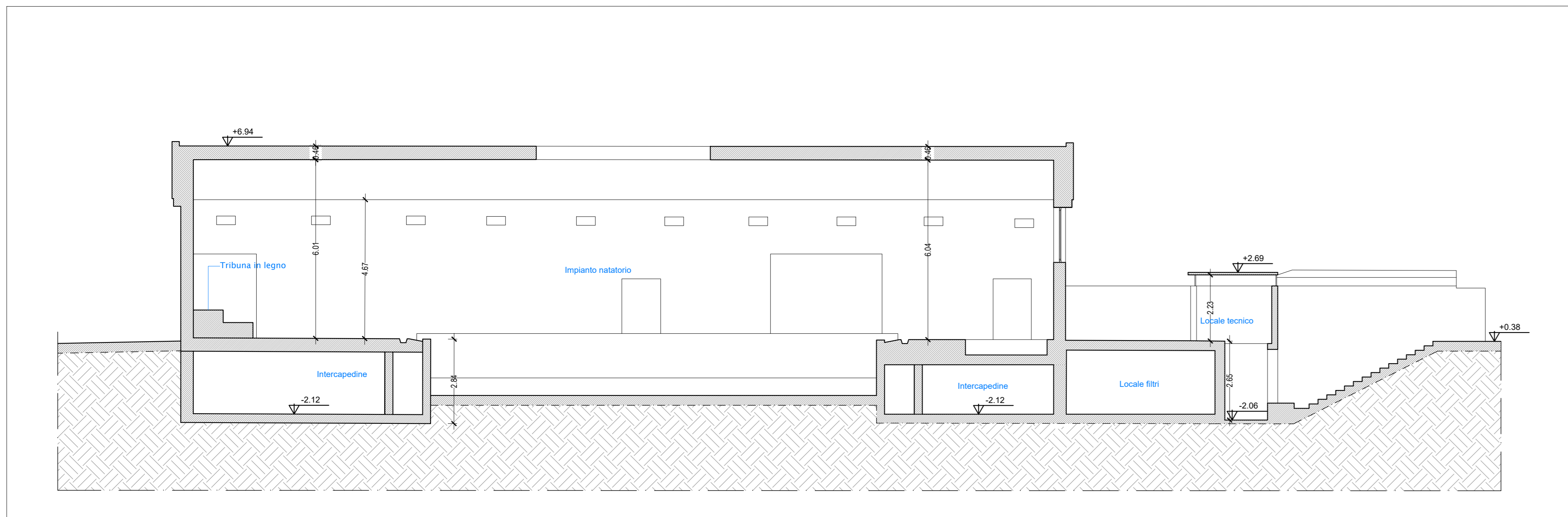
Sezione B-B' - scala 1:100
