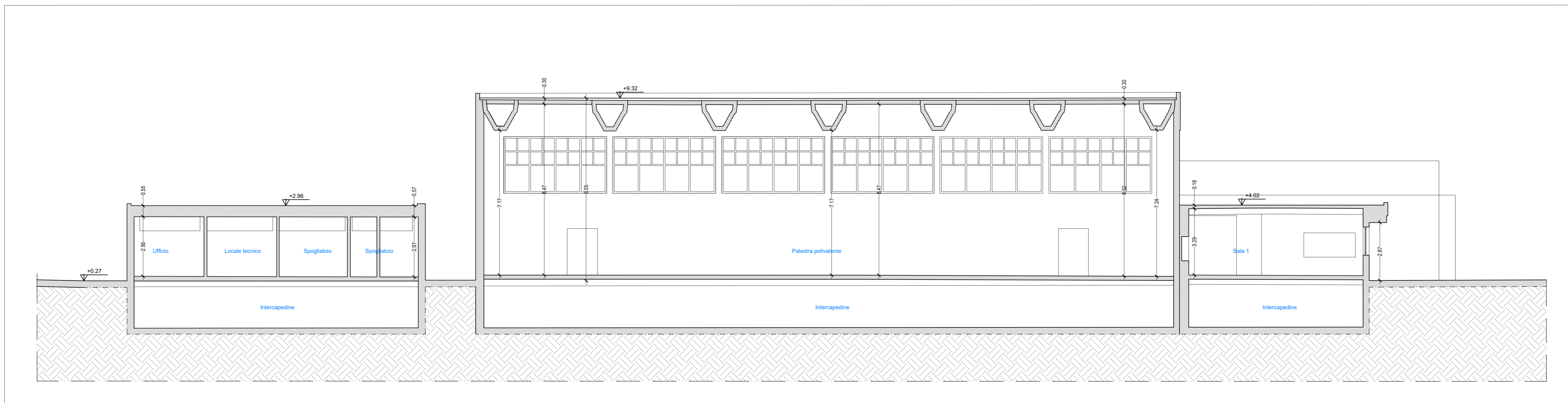
Sezione C-C' - scala 1:100
