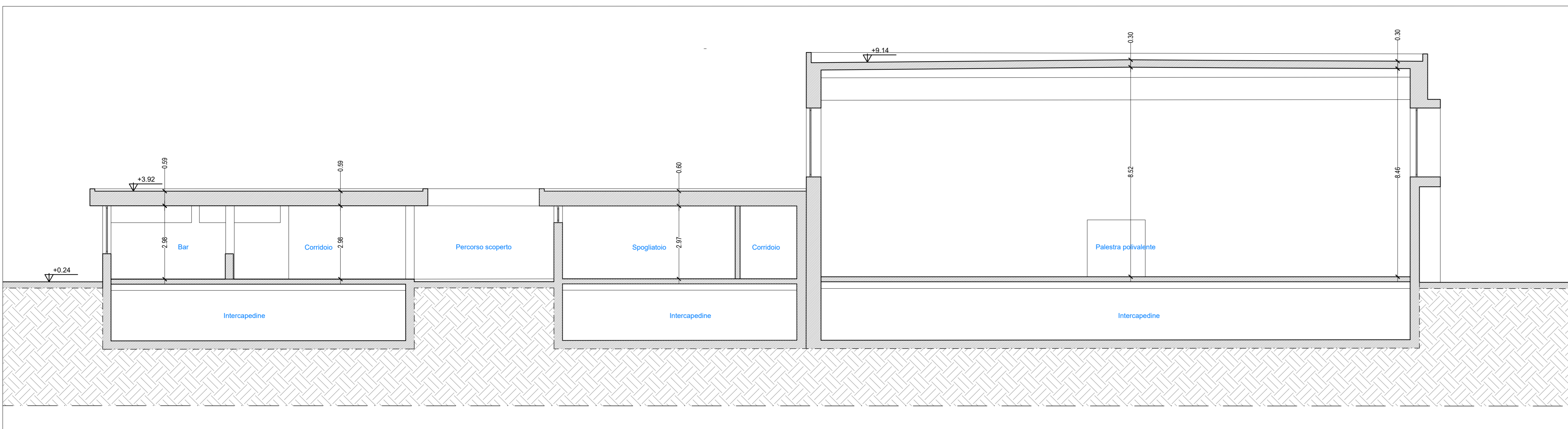
Sezione D-D' - scala 1:100
