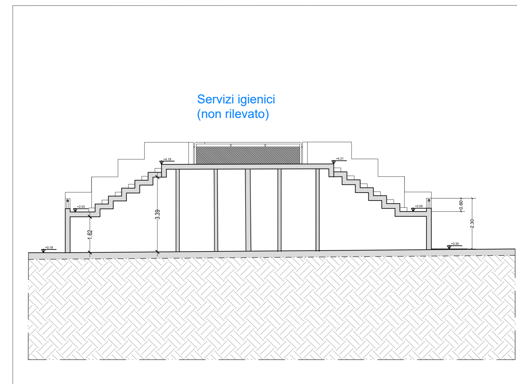
Sezione E-E' - scala 1:100
